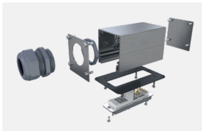
Рис.3. Состав защитного корпуса
